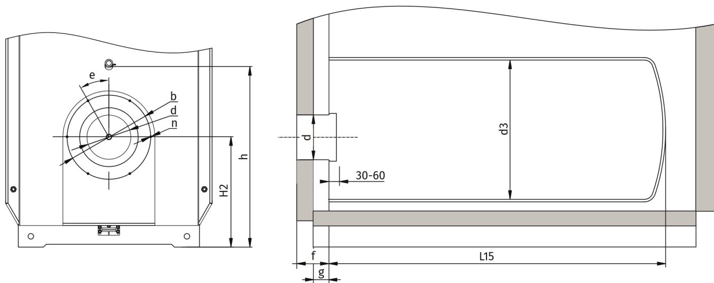
Рисунок 3 - Размеры присоединения горелки
