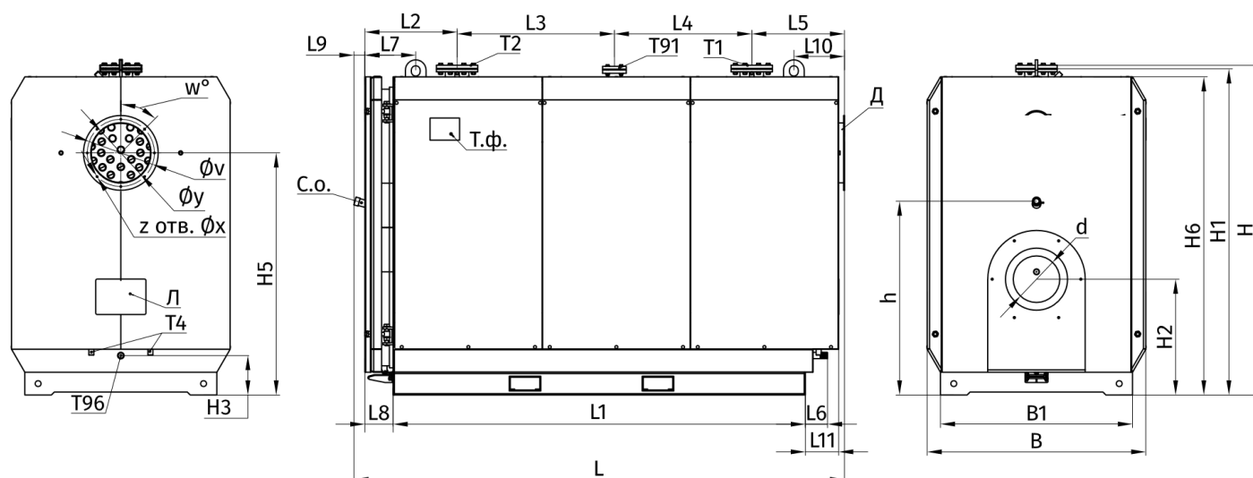
Рисунок 1 - Габаритные размеры
